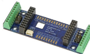
51971 adapterprint LokSound / LokPilot L met schroefaansluitingen
